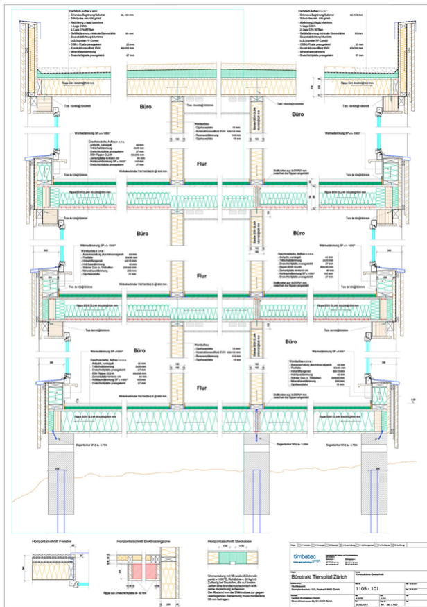
Querschnitt Gebäude
