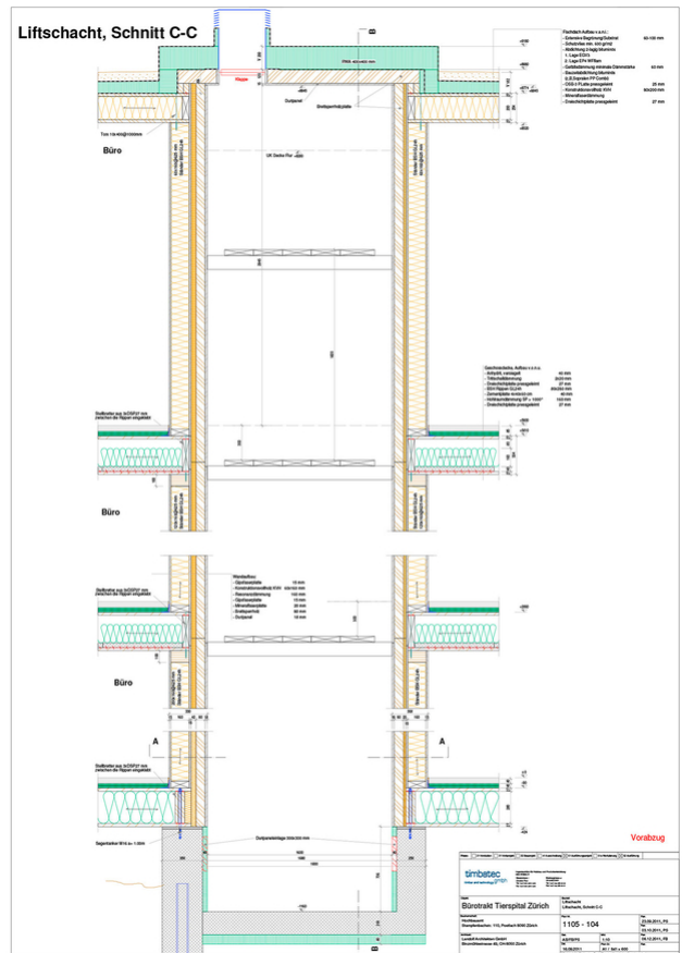
Schnitt durch Liftschacht
