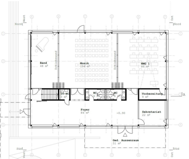
Grundriss Mehrzweckraum
