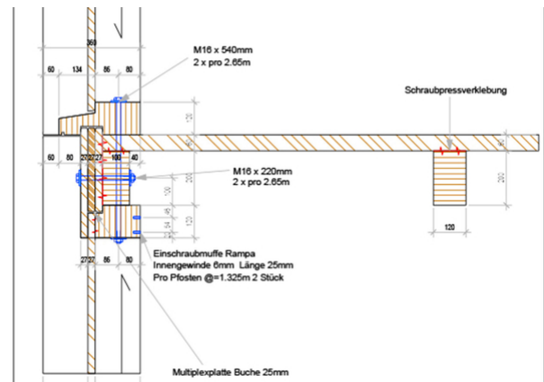
Anschlussdetail: Aussenwand-Geschossdecke
