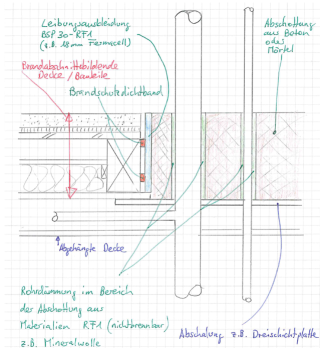
Systemskizze Abschottungen
