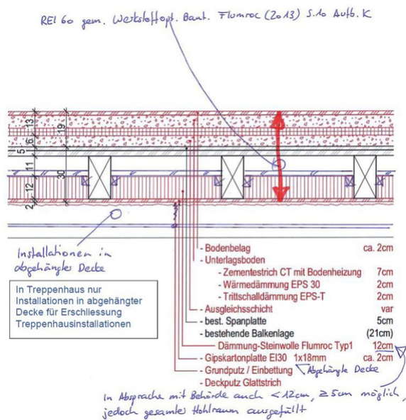
Systemskizze Ertüchtigung
