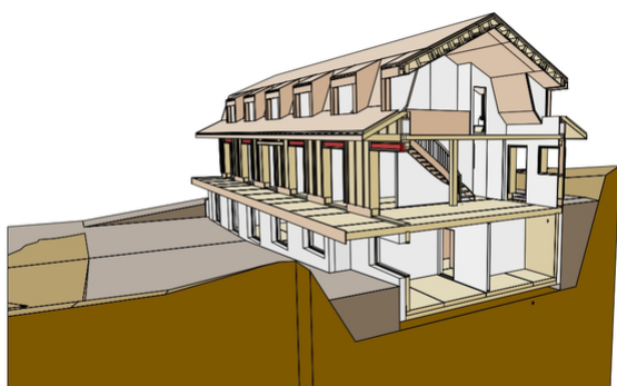
Coupe du bâtiment
