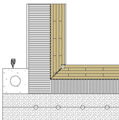
Détail de la cave en bois
