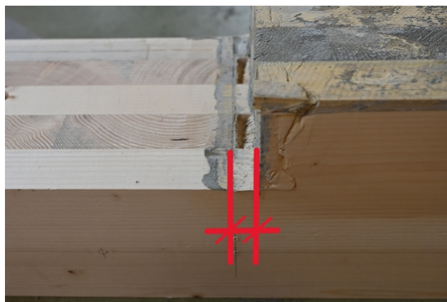
Comportement ductile de la came de cisaillement en CLT sur l'éprouvette (lors des essais réalisés à l'ETH Zurich)
